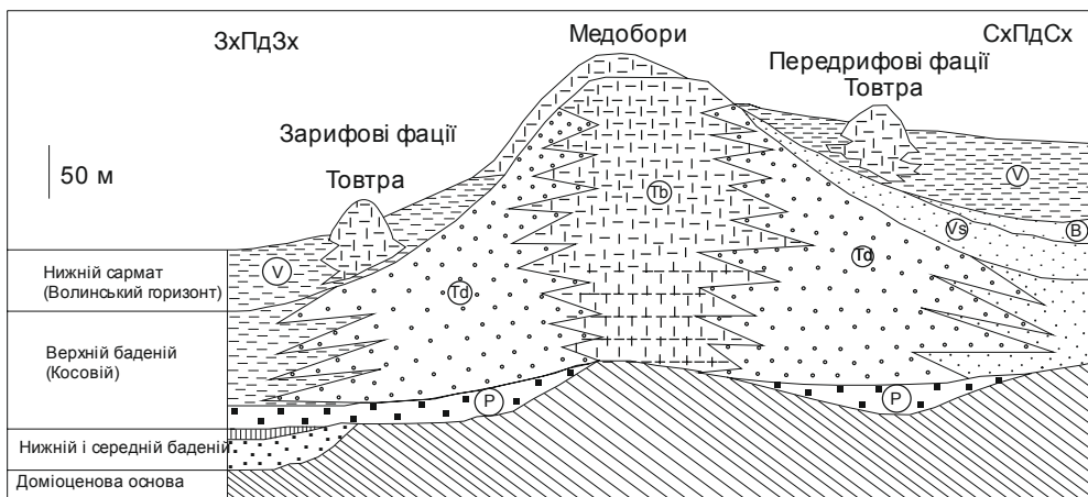
Рис. 3. Схематична геологічна (структурна і вікова) модель будови біогермів Медобори (поперічний розріз). Просторове співвідношення біогермних фацій пасма Медоборів і Товтра, деталі їх літології і головних структурно-літологічних одиниць
