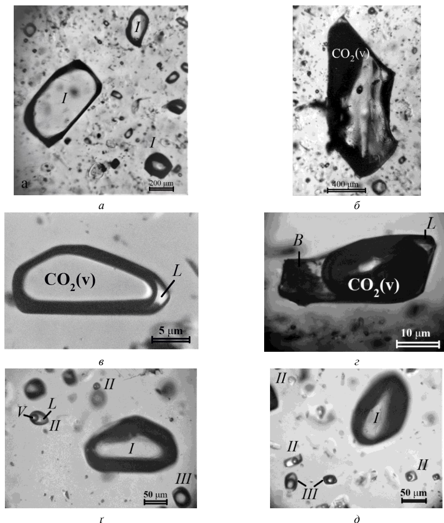
Рис. 4. Первинні флюїдні включення, що прилипли до грані ромбоєдра моріону (а–б), і сингенетичні первинні включення \text{CO}_2 -флюїду й водного розчину (г, д): I – включення \text{CO}_2 -флюїду; II – газиво-рідкі включення ( L \sim 80 об. %); III – включення гетерогенного наповнення; L – водний розчин; \text{CO}_2(V) – \text{CO}_2 -флюїд (газова фаза); B – тверда фаза.
