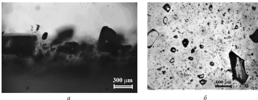
Рис. 3. Первинні включення CO 2 -флюїду в кварці пізньої генерації, розташовані безпосередньо на грані ромбоєдра моріону у площині, паралельній до граней призми {1120} (а) і ромбоєдра (б).
